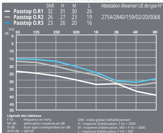
COURBES D'ATTENUATIONS
